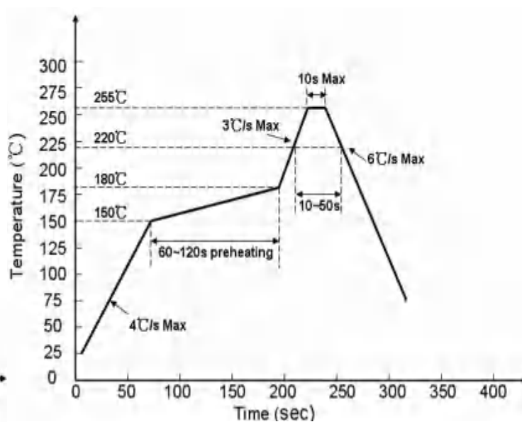
无铅焊接
