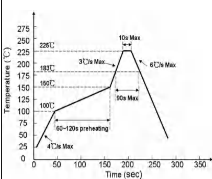
有铅焊接
