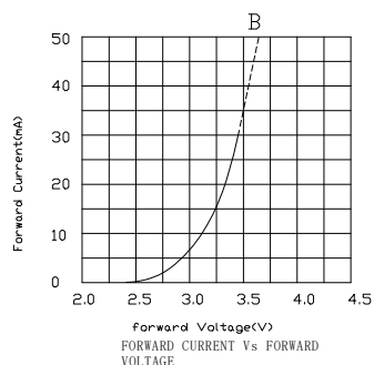
正向电流与正向电压关系曲线图
