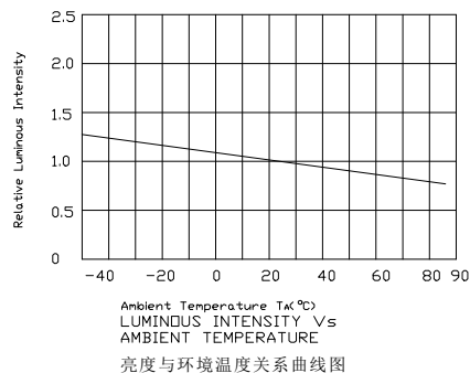
亮度与环境温度关系曲线图
