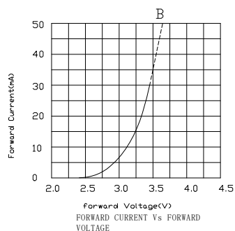
正向电流与正向电压关系曲线图
