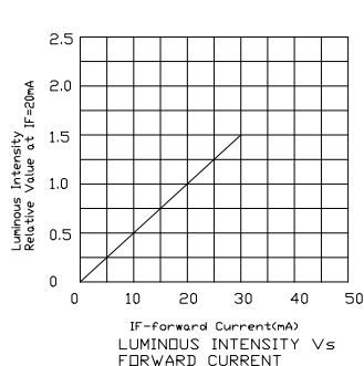
亮度与正向电流关系曲线图
