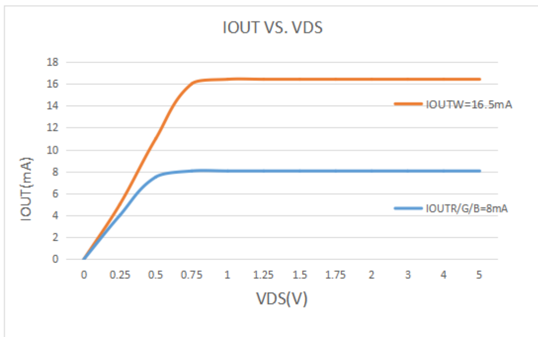
Fig. MW1877A I_{OUT} 与 OUT 端口电压 V_{DS} 的关系图
