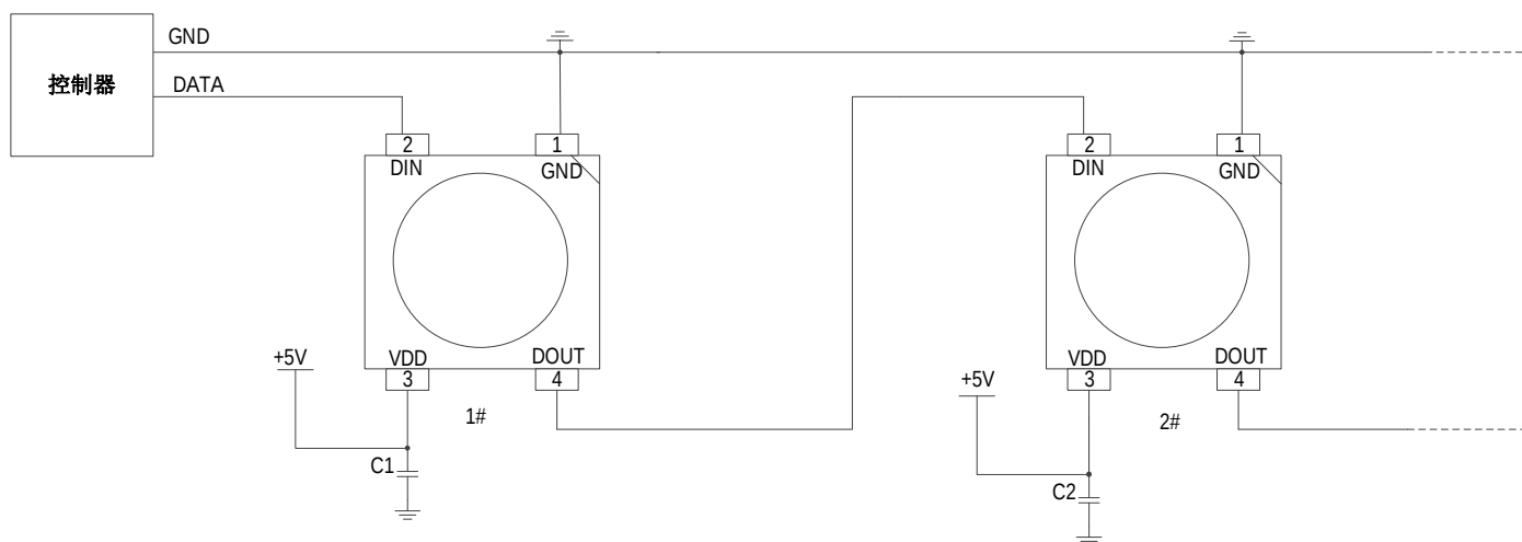
Fig. MW1877A 产品应用示意图
