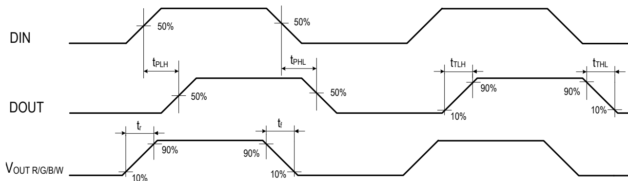
Fig. MW1877A 动态参数测试示意图
