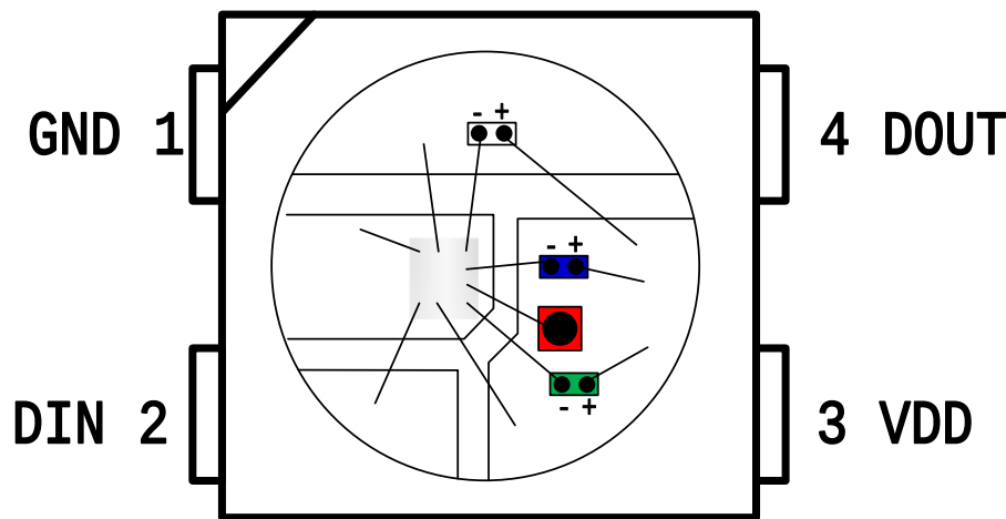
Fig. MW1877A 封装打线参考示意图
