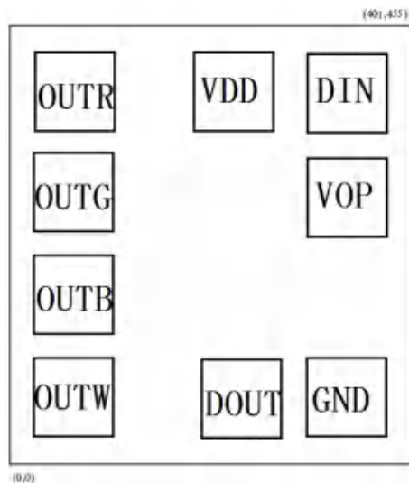
Fig. MW1877A PAD 图
