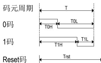
Fig. MW1877A 归零码数据通信协议图
